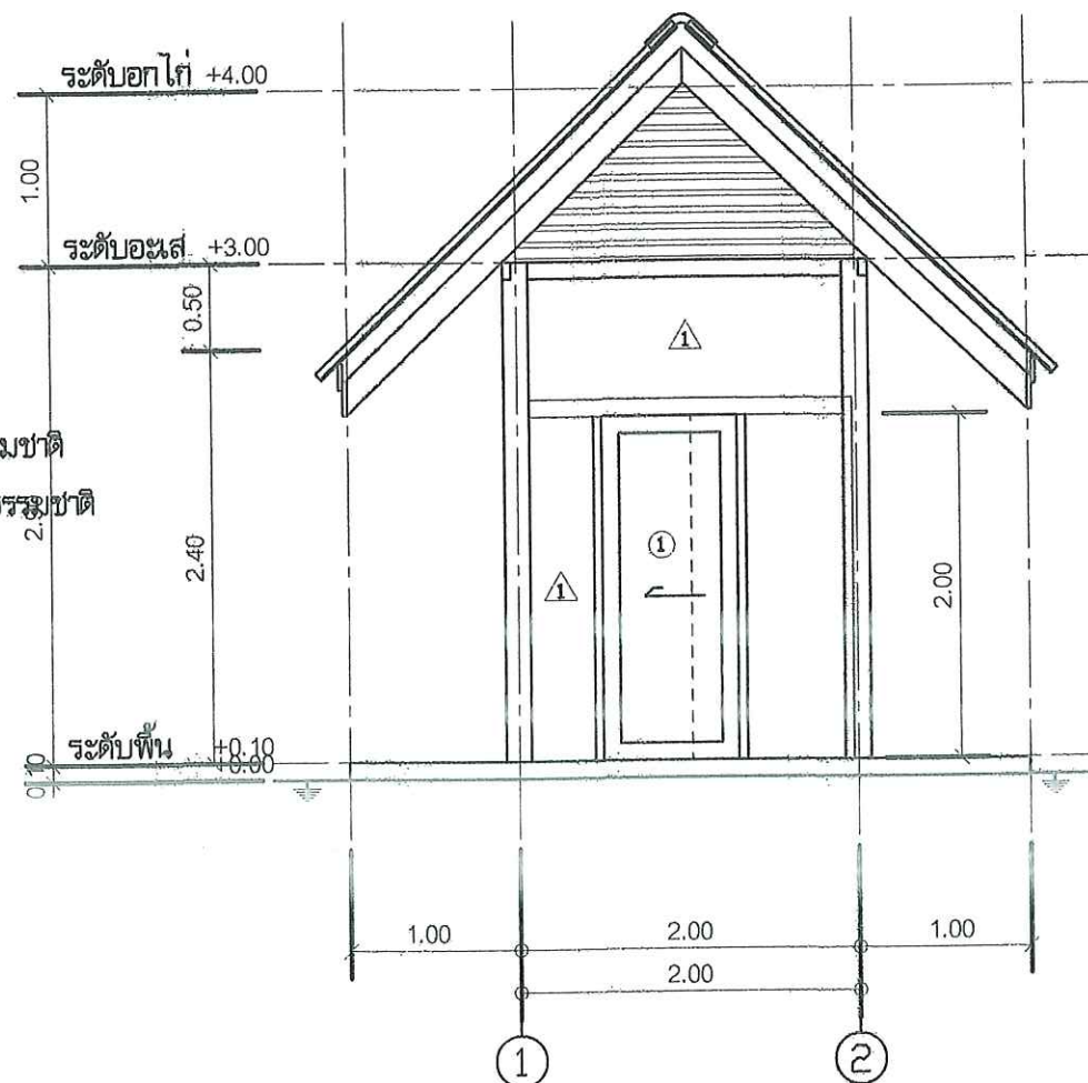
รูปตัด 1-1 มาตราส่วน 1 : 50
