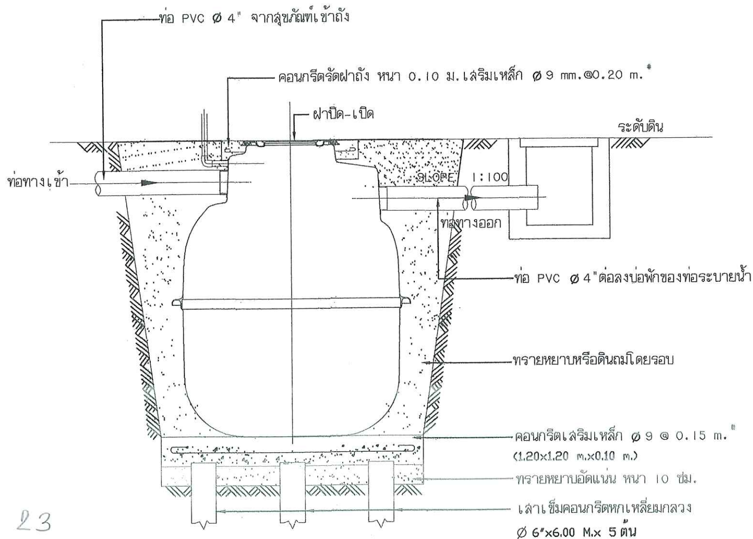
แบบขยายบ่อบำบัดน้ำเสียสำเร็จรูป
