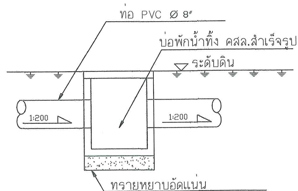
ขยายรูปตัด 2-2 มาตรฐาน 1 : 25
